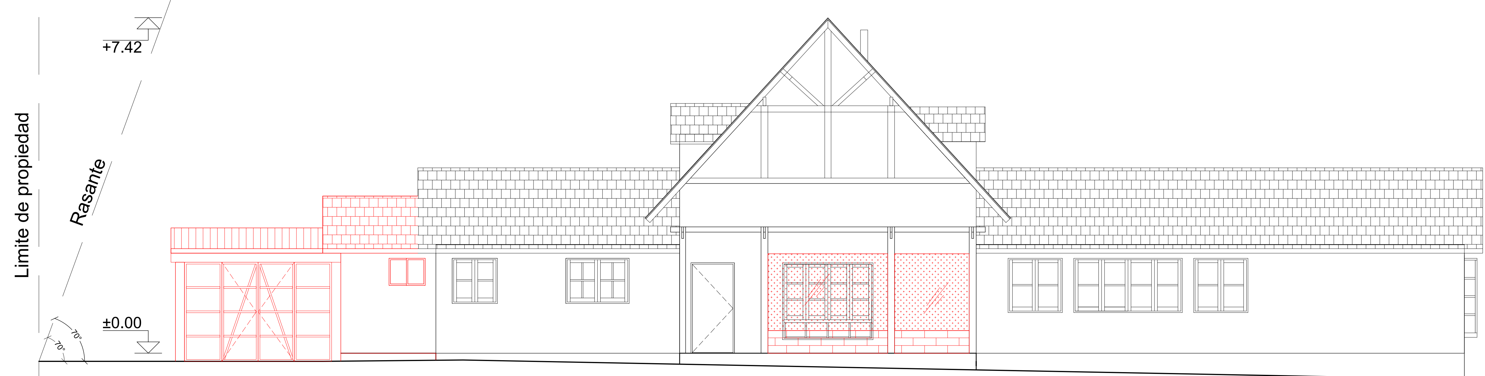
Elevación Sur Esc 1:50
