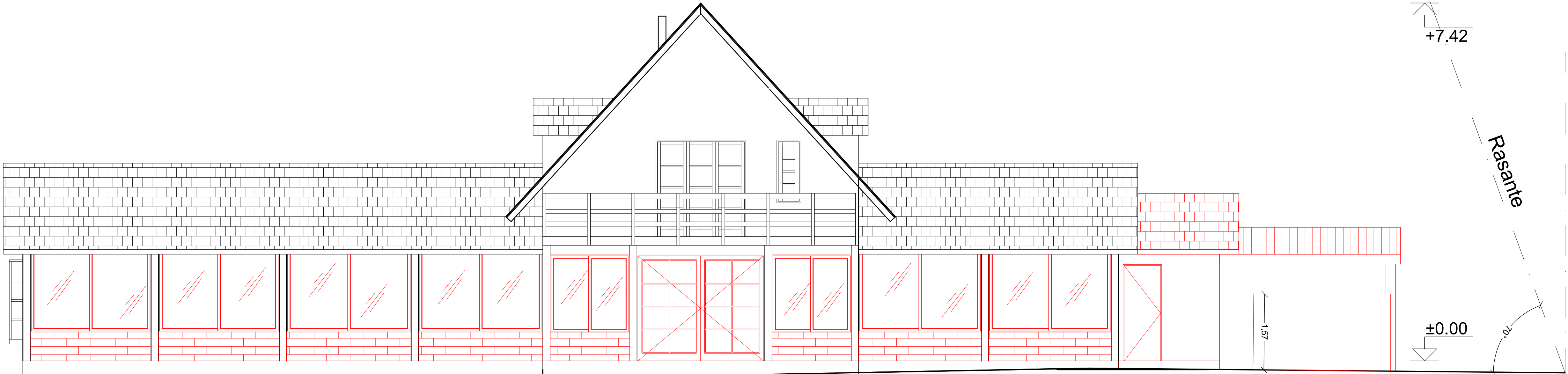
Elevación Norte Esc 1:50
