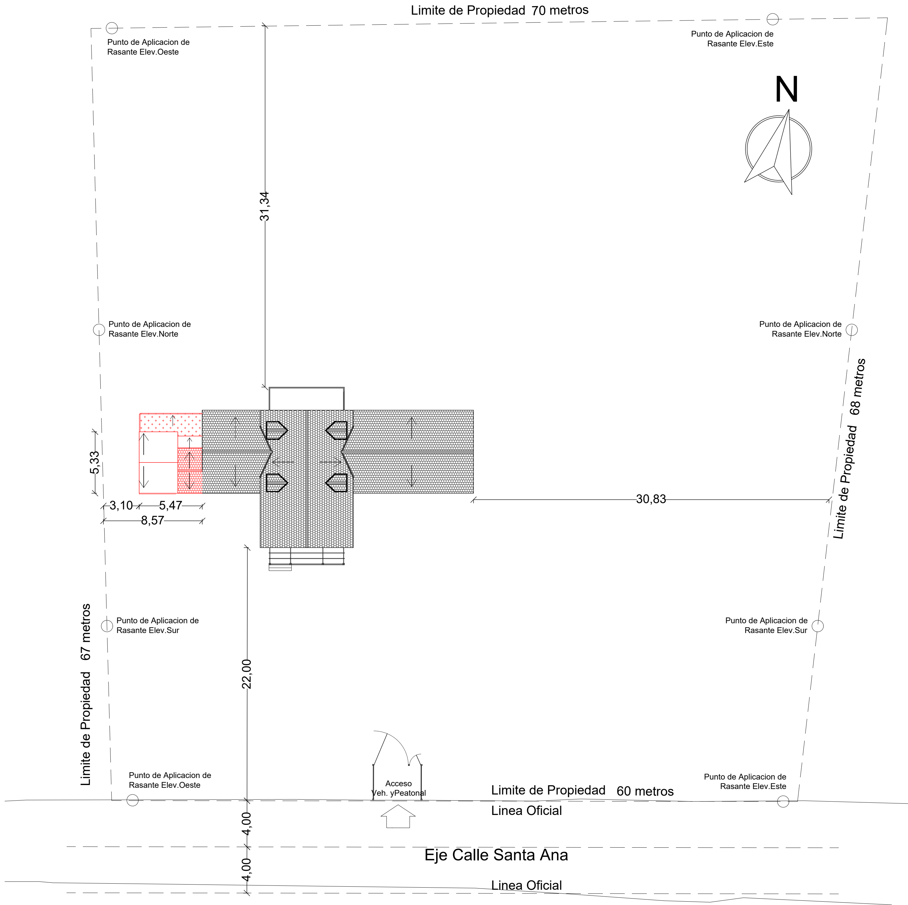
Planta Emplazamiento Esc 1:200
